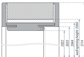
▼ ADJUSTABLE 80 DOOR FRAME
